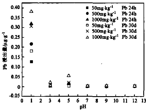
图 4 滤料中 Pb 浸出量与 pH 的关系
