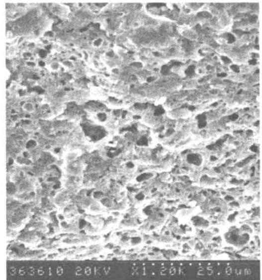
图 6 滤料表面的电镜照片(1000℃)
