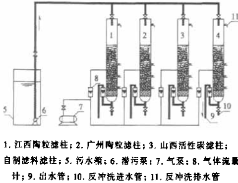
图7 BAF试验装置
