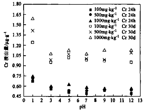
图 2 滤料中 Cr 浸出量与 pH 的关系
