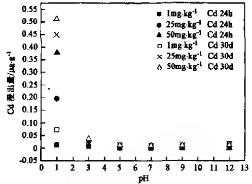
图 1 滤料中 Cd 浸出量与 pH 的关系
