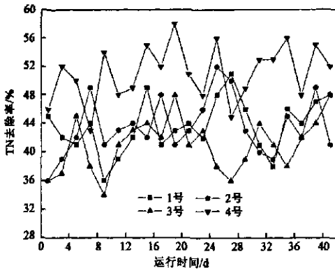
图 11 4种滤料 TN 去除率比较
