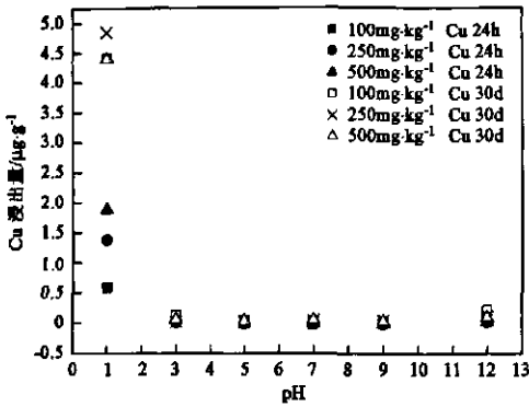
图 3 滤料中 Cu 浸出量与 pH 的关系
