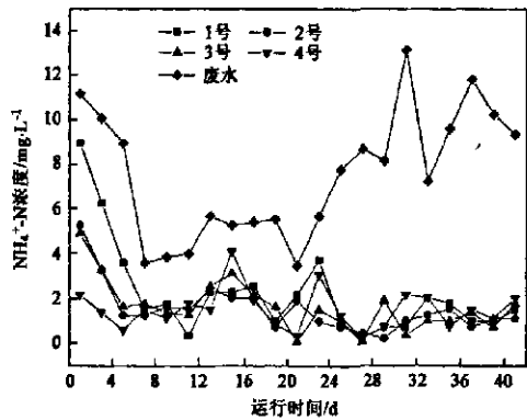
图10 4种滤料 NH 4 + -N 去除率比较
