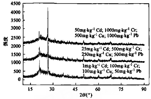
图 5 滤料 XRD 分析(1000℃)
