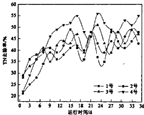
图9 4种滤料 TN 去除率比较
